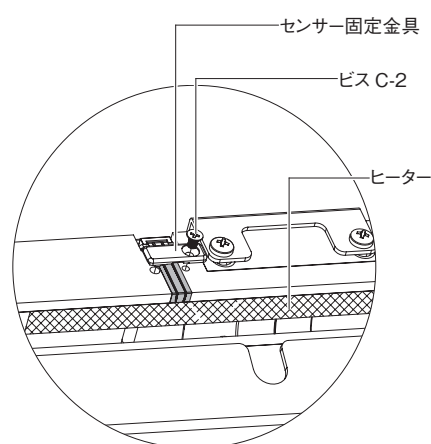
接続コネクタ部の拡大イラスト
