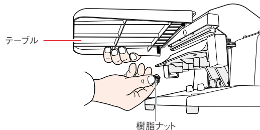
樹脂ナット
